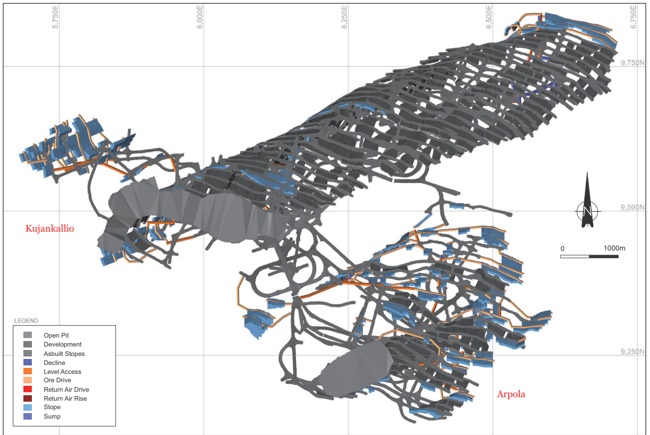
Figure 3 – Jokisivu Mine Design. Plan View.
